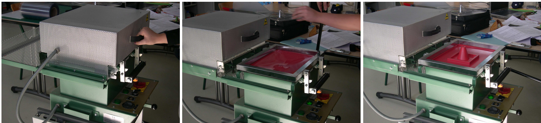
Etapes de thermoformage
